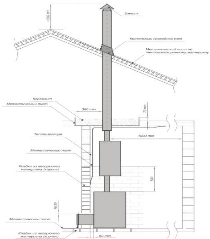
Рисунок 1. Установка печи. Вид сбоку
