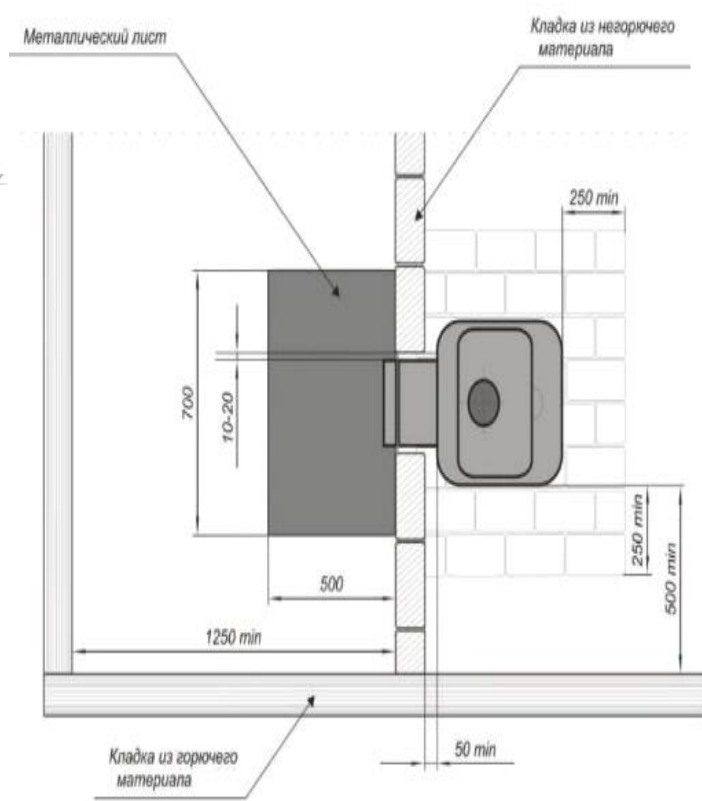
Рисунок 2. Схема установки печи. Вид сверху
